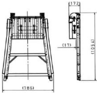
収納状態図
